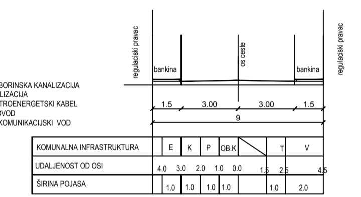
KARAKTERISTIČAN POPREČNI PRESJEK A M 1:200
